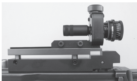
Figura 20: supporto dell'alzo per il F ass 57 per il montaggio di comuni alzi circolari resistente ai contraccolpi – rinculo, diversi modelli
